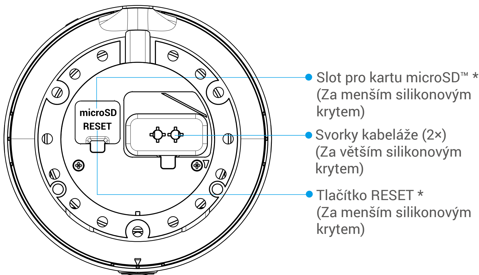
Pohled zespodu
